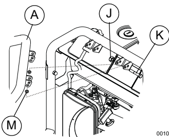
Figura 2-10. Asa de transporte
