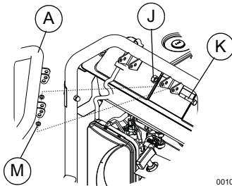
Figure 2-10. Montage de la poignée
